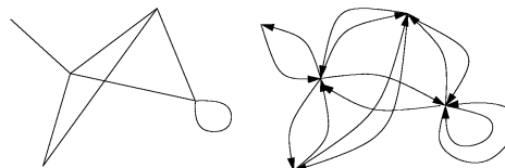
Figuur 1 Een graaf X (links) en de bijbehorende geïoriënteerde graaf X^+ (rechts)
